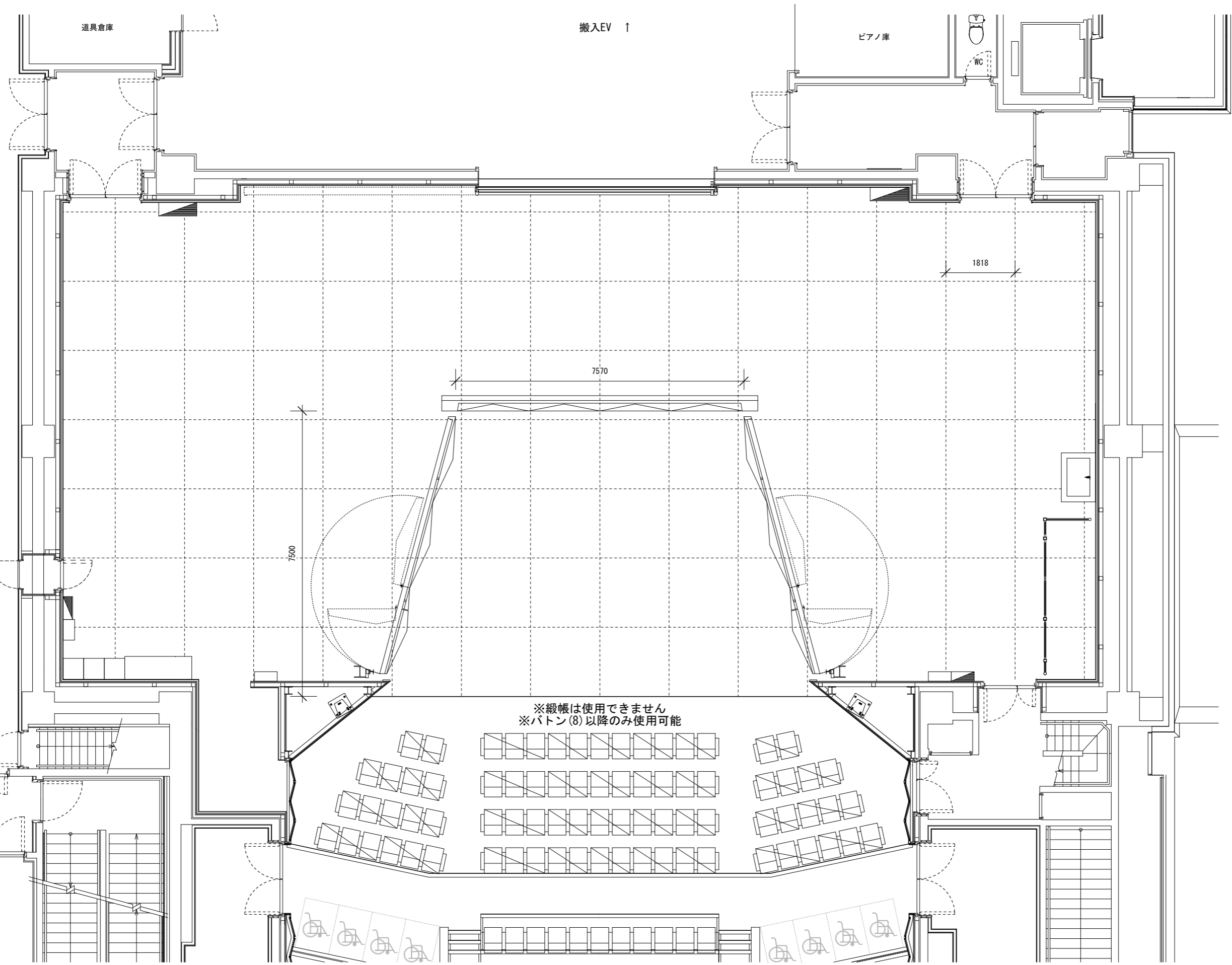
サンポートホール高松 第1小ホール音響反射板舞台平面図 A3:1/100
