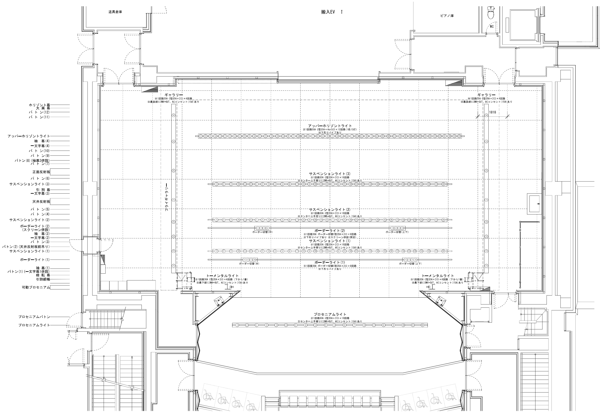
サンポートホール高松 第1小ホール照明吊物コンセント図 A3:1/100
