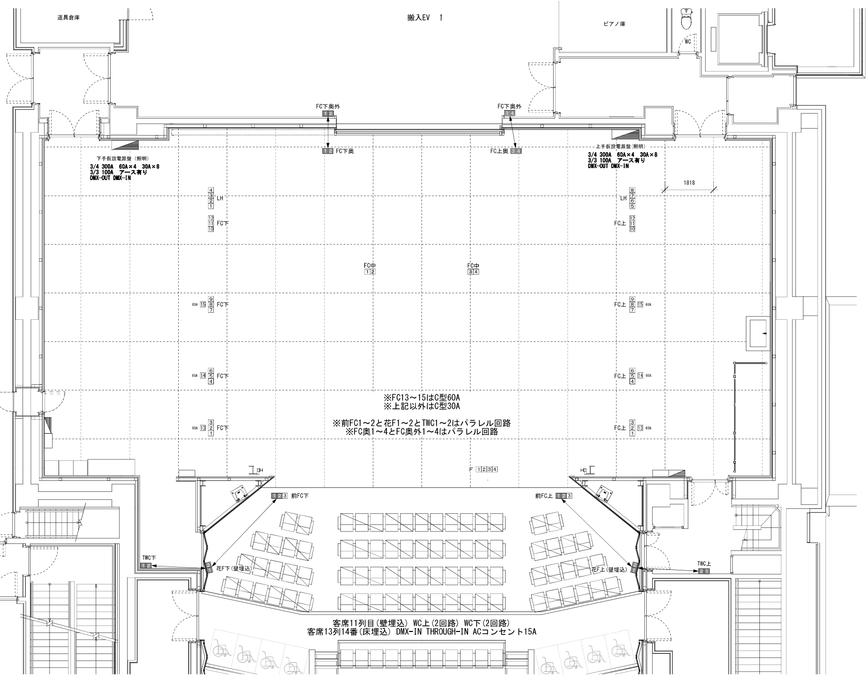
サンポートホール高松 第1小ホール照明床面コンセント図 A3:1/100
