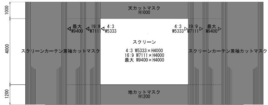
正面図
