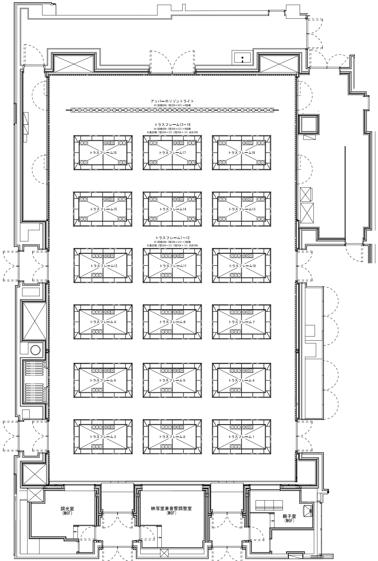
サンポートホール高松 第2小ホール照明吊物コンセント図 A3:1/100
