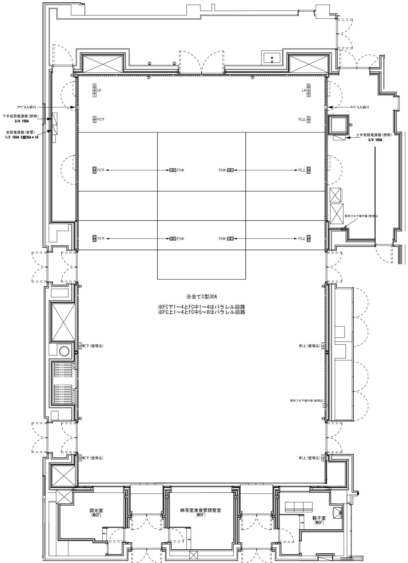
サンポートホール高松 第2小ホール照明床面コンセント図 A3:1/100
