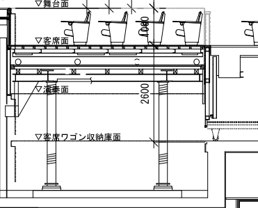
サポートホール高松 大ホール舞台断面図 A3:1/100
