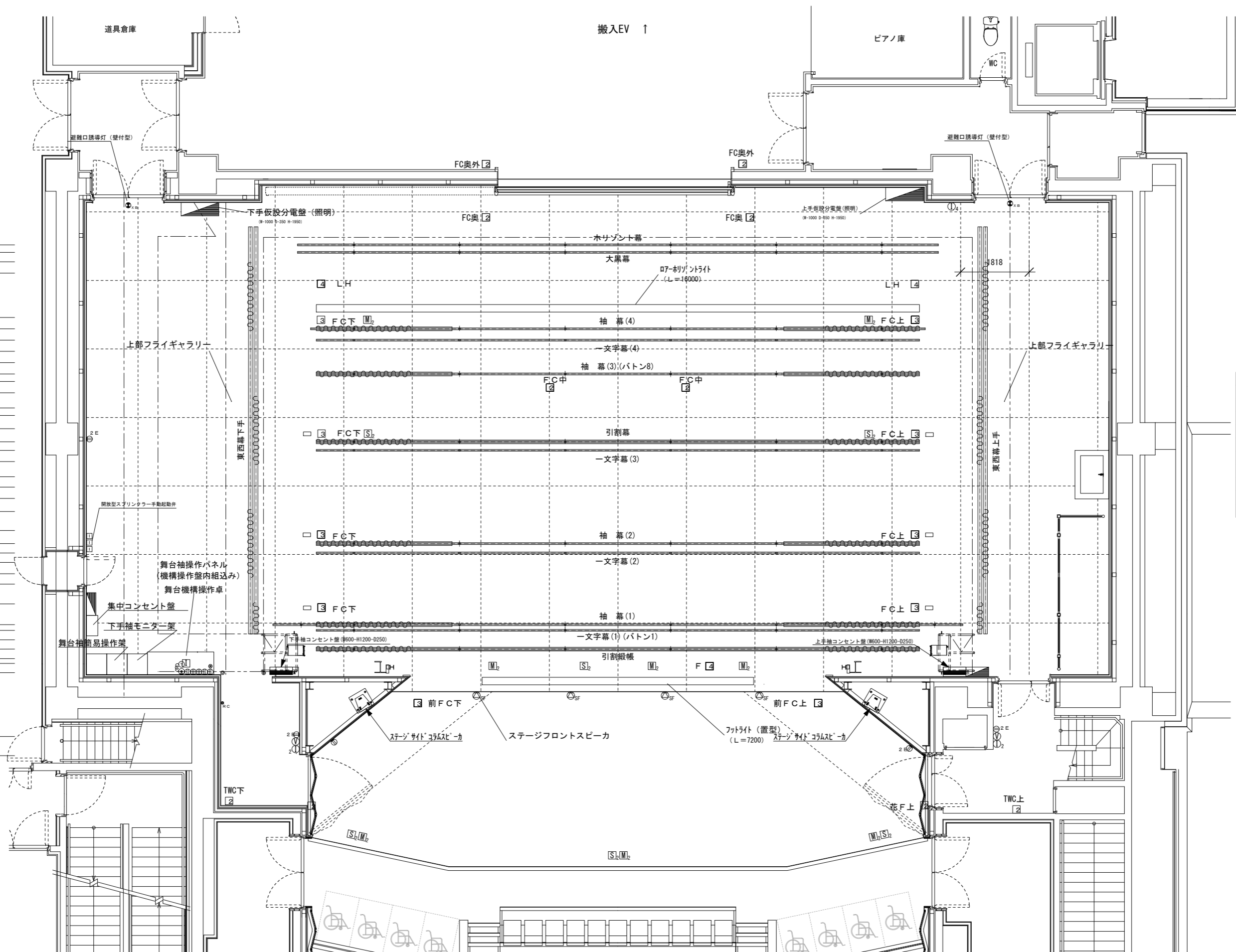
サンポートホール高松 第1小ホール主要設備詳細図 A3:1/100
