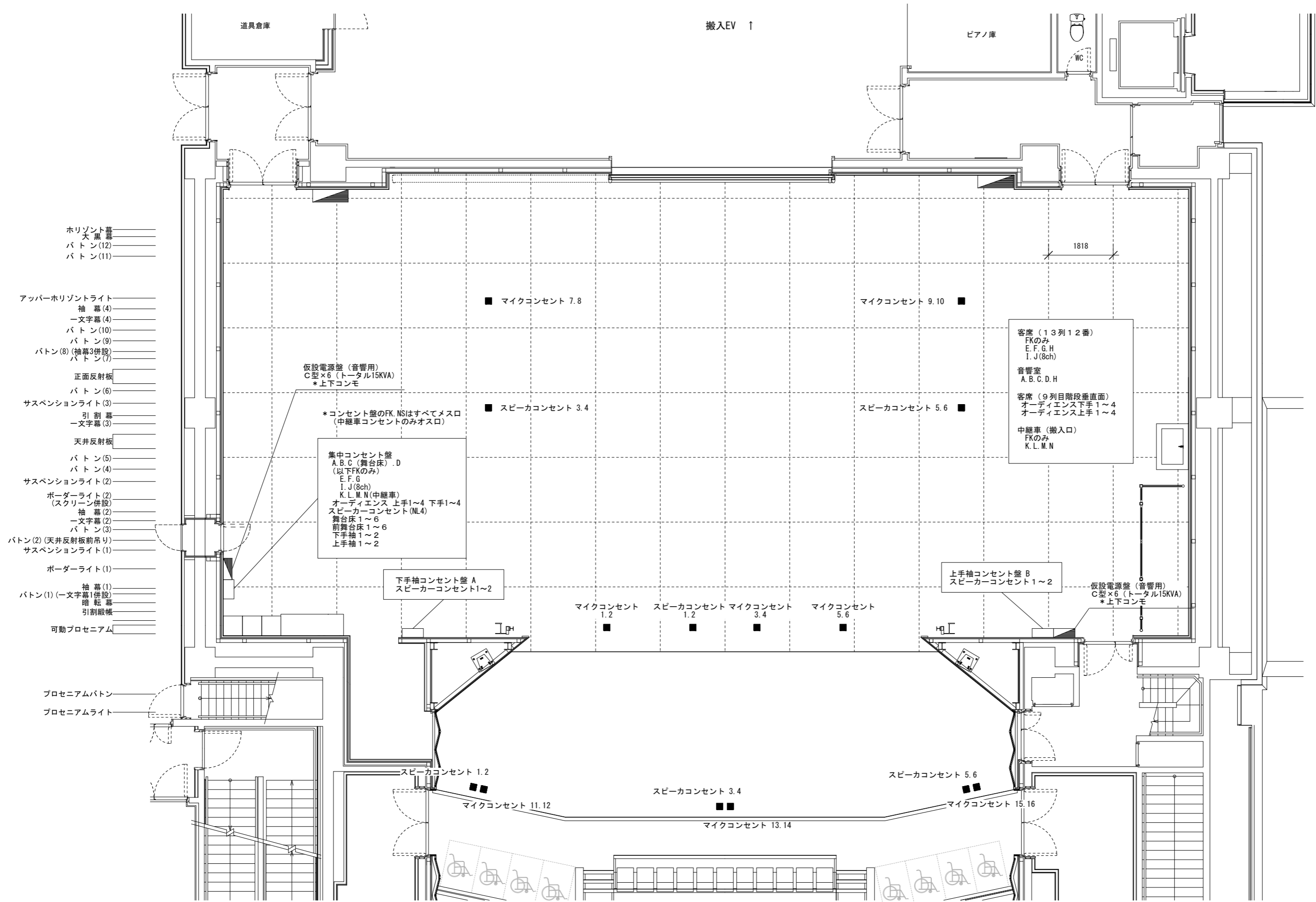
サンポートホール高松 第1小ホール音響コンセント図 A3:1/100
