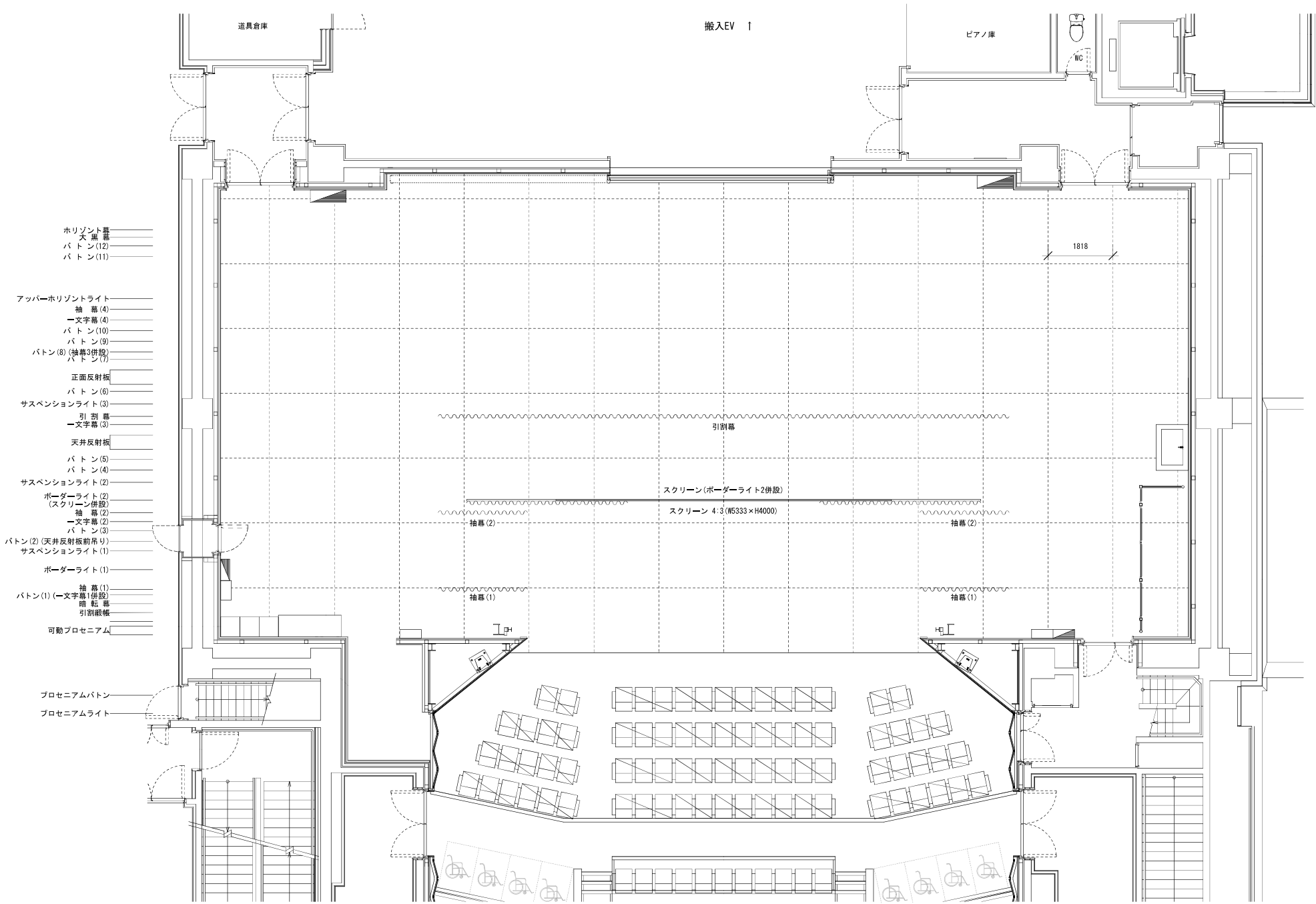
サンポートホール高松 第1小ホールスクリーン使用平面図 A3:1/100
